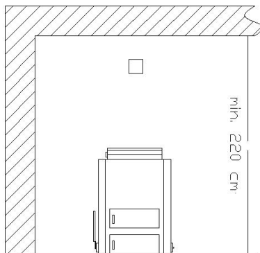
Rys. Usytuowanie kotła
