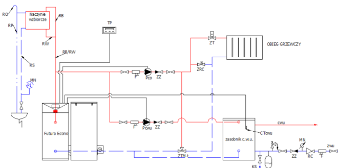
Poglądowy schemat instalacji c.o. i c.w.u z termostатыcznym zaworem 3-drogowym
