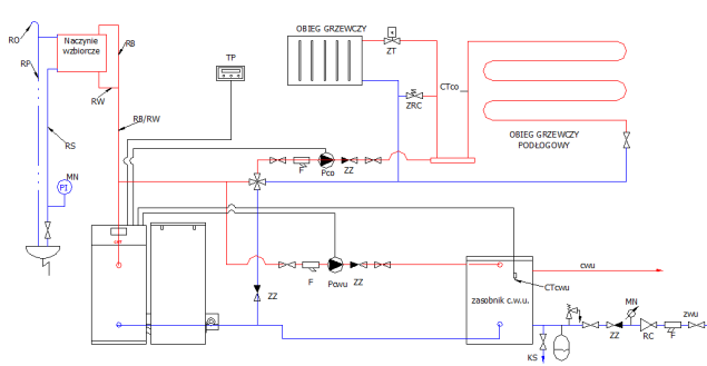
Poglądowy schemat instalacji c.o. z zaworem 4 drogowym
