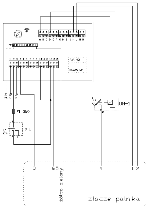
Schemat podłączenia palnika do regulatora RK2006LP
