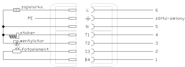
Złącze elektryczne palnika
