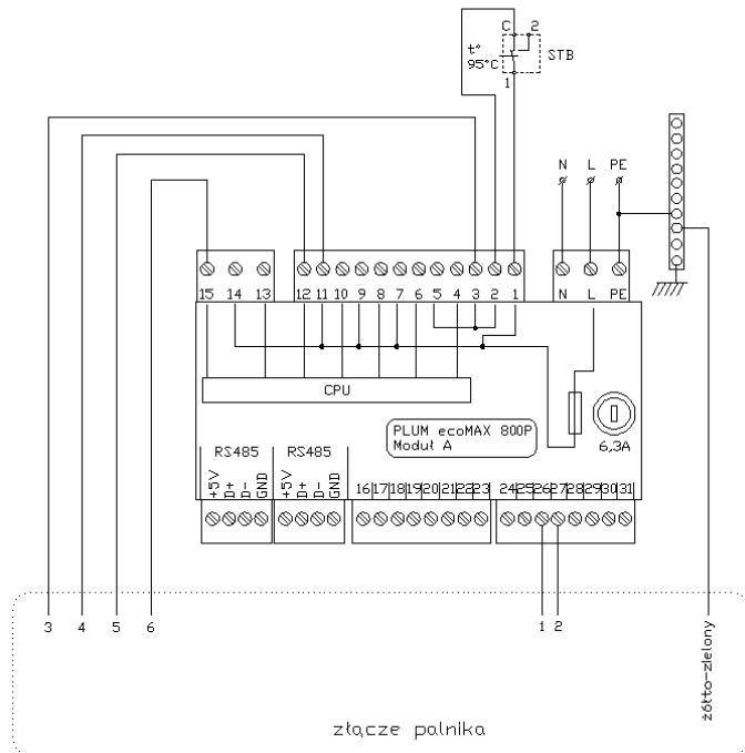
Schemat podłączenia palnika do regulatora ecoMAX 800P
